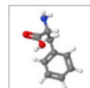
molecole.png
